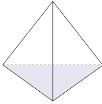
각뿔
