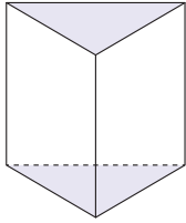
각기둥
